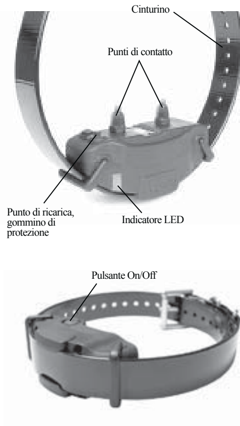
Collare Ricevitore
