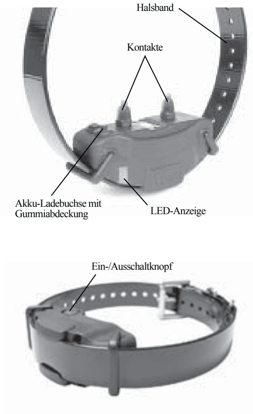
Empfängerhalsband
